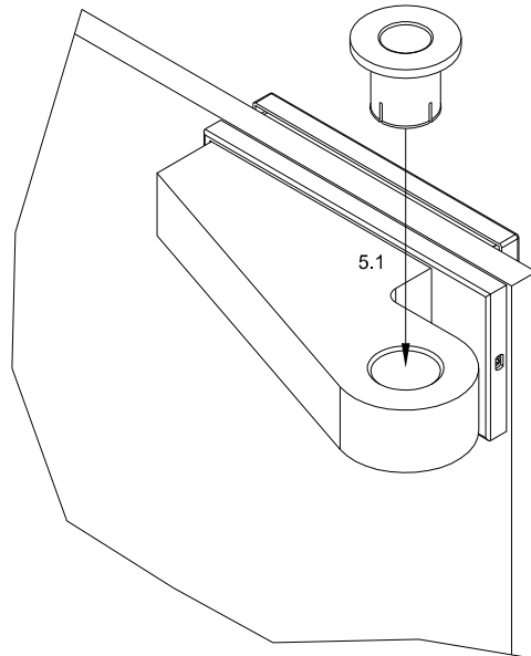
Oberer Eckbeschlag Top patch fitting
