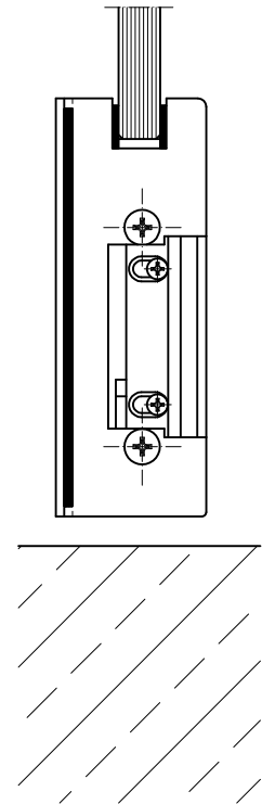
Türschiene mit E-Öffner (Seitenteilschiene) (Ausf. rechts)
